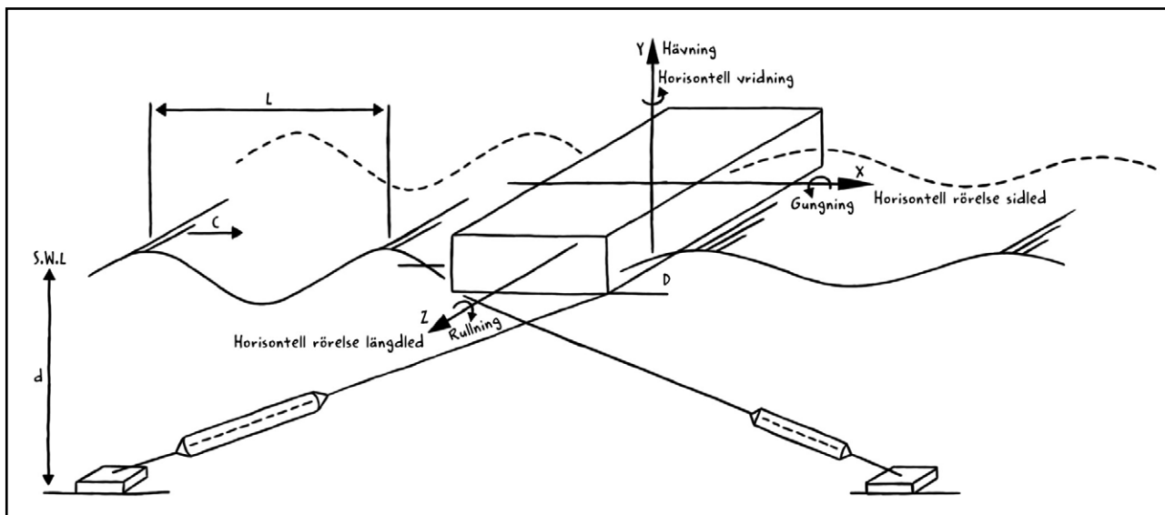
Fig. 2:15 Vågbrytande ponton.
