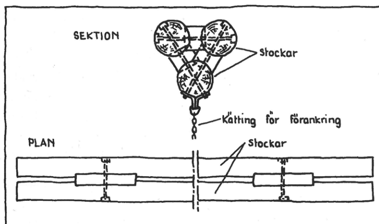
Fig. 2:8 Stocklänsa.
