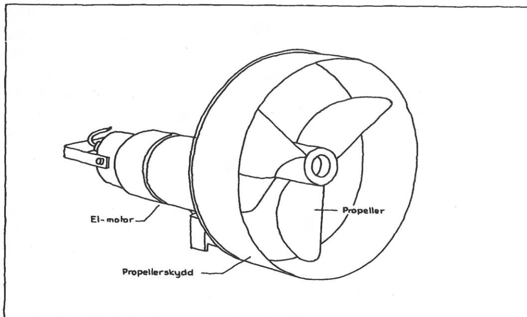
Fig. 2:41 Isbegränsningsanläggning. Strömbildare.
