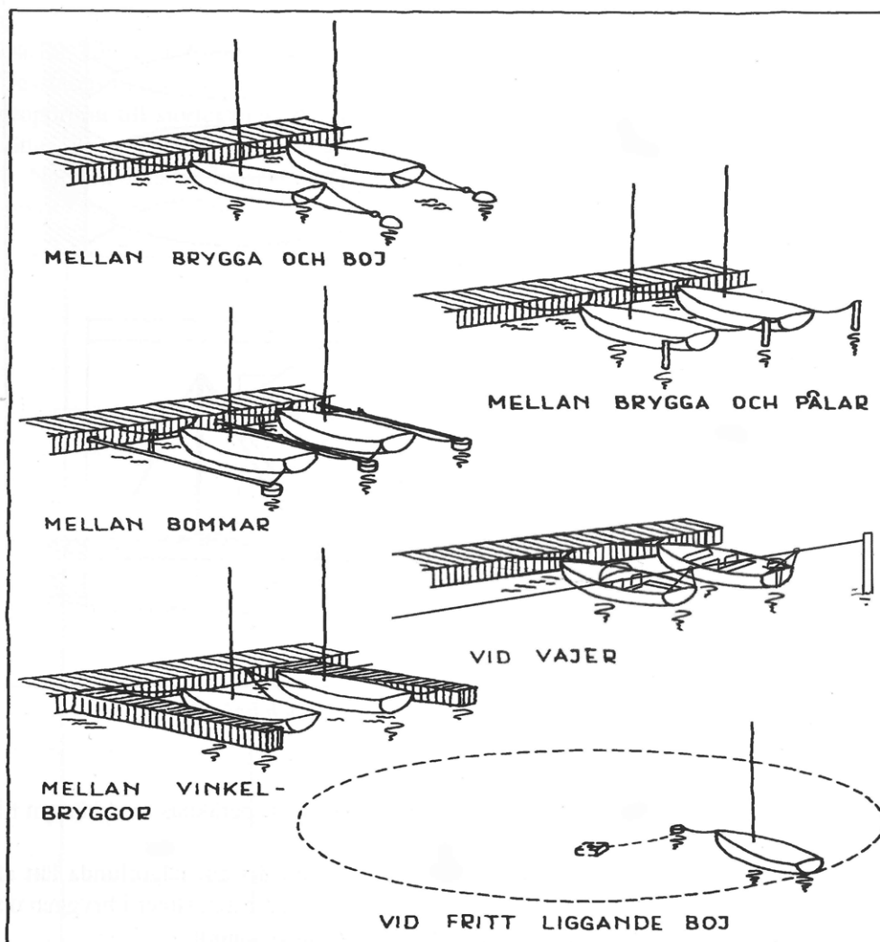
Fig. 2:27 Översikt, förtöjningsätt.
